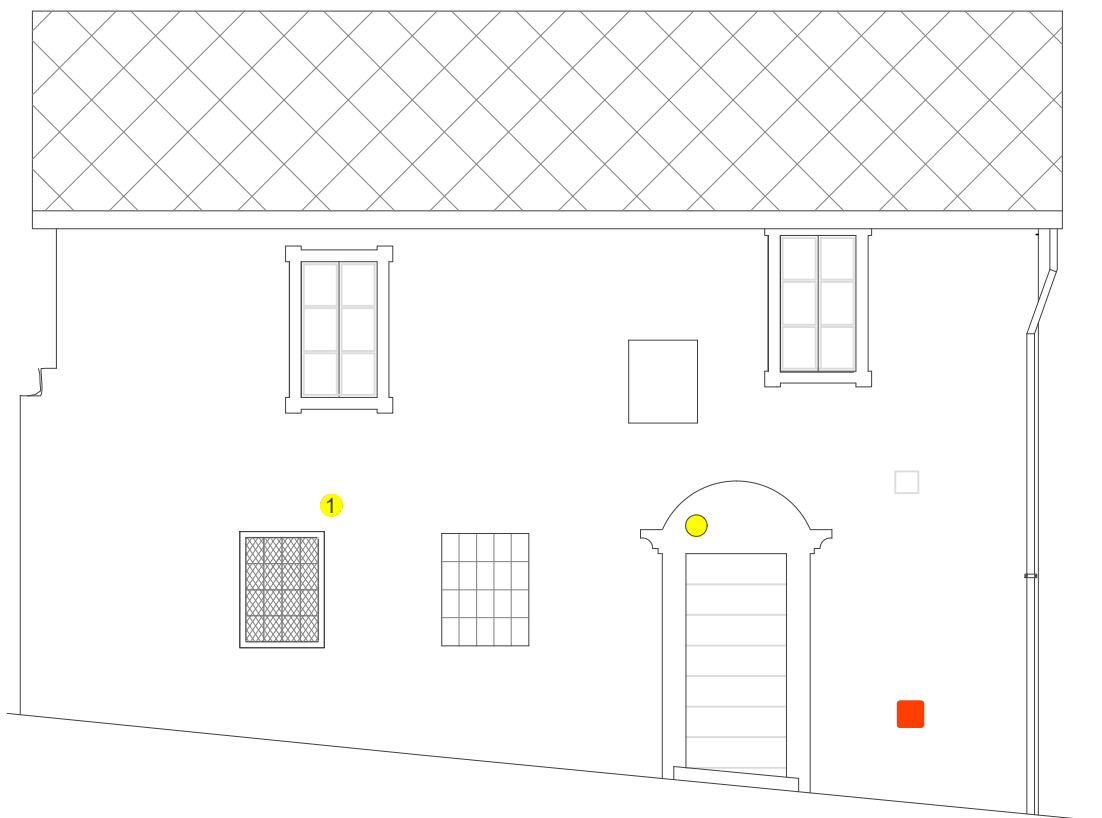
PROSPETTO FRONTE STRADA
