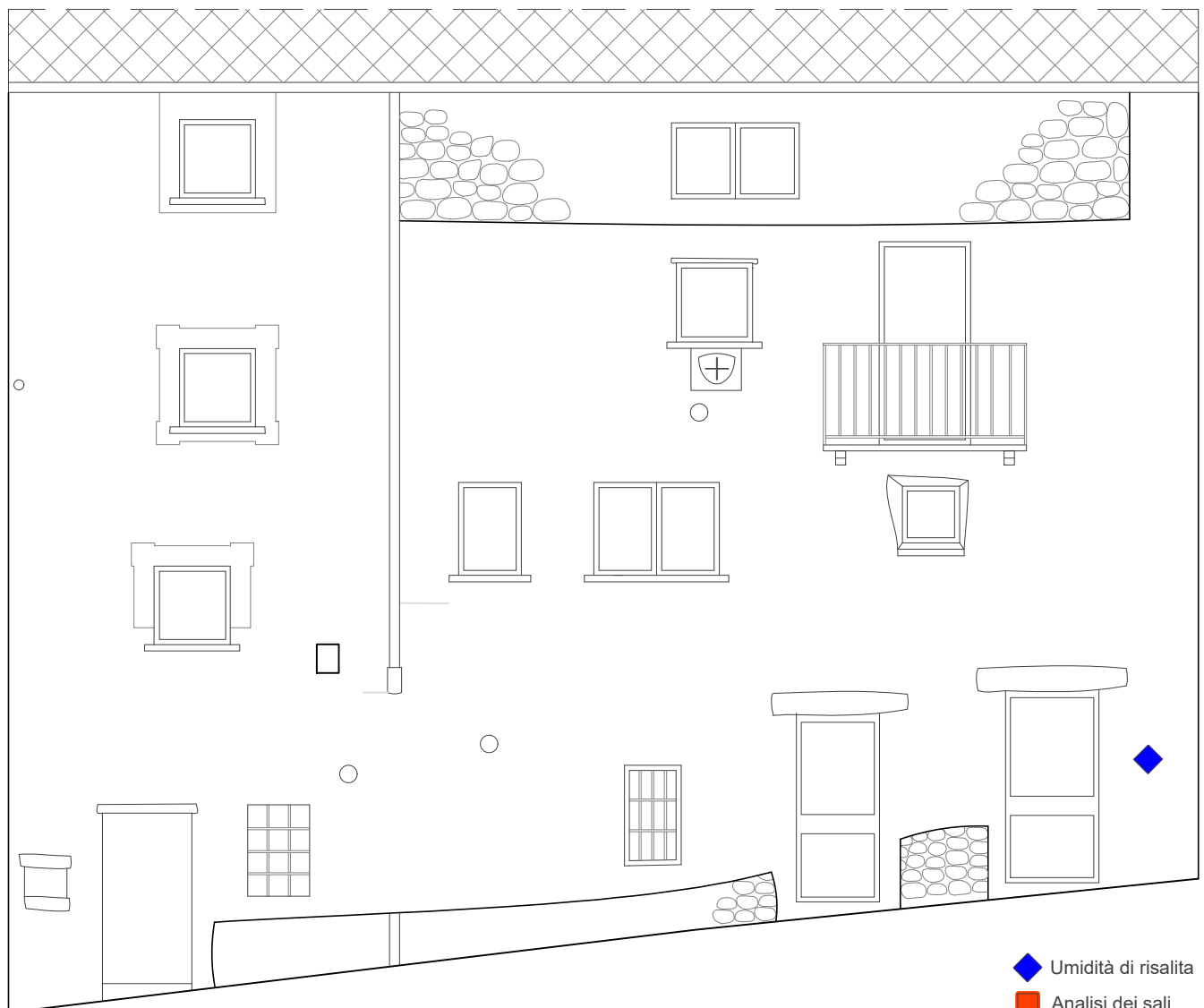
PROSPETTO FRONTE STRADA
