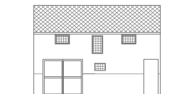
PROSPETTO FUORI SCALA
