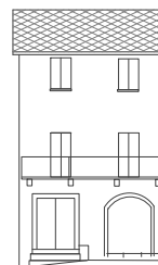
PROSPETTO FUORI SCALA
